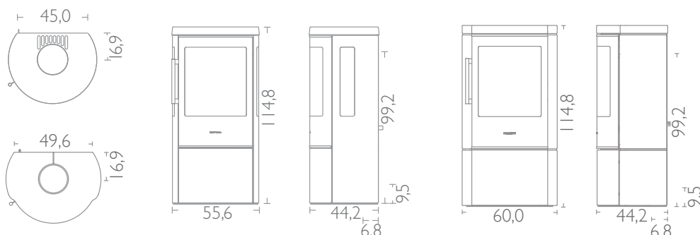
HWAM 3630c met zijruiten
