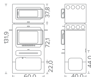
HWAM Classic 4 met oven en houtvak
