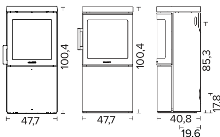
HWAM 3120c met style handgreep, roestvrij staal
