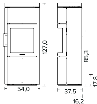
HWAM 3520m met speksteen
