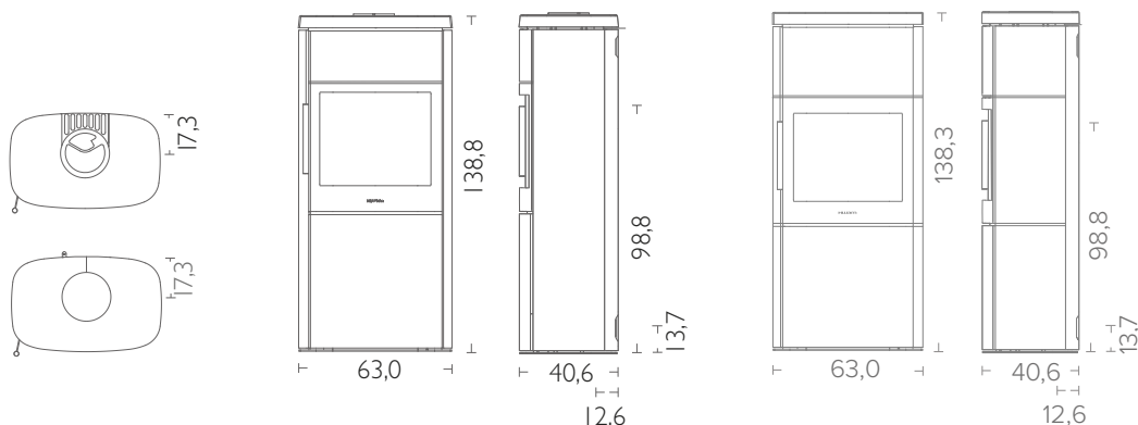
HWAM 4660m met Tobacco
