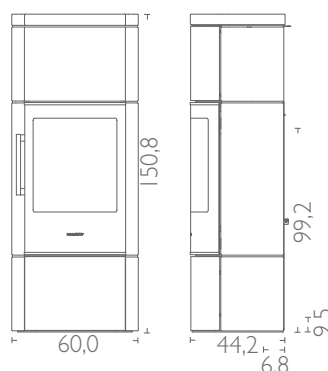
HWAM 3660m met speksteen
