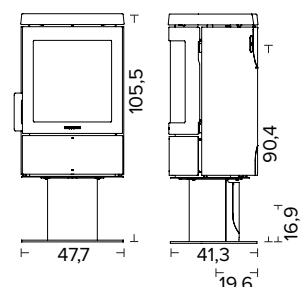
HWAM 3110c met voetstuk en style handgreep, zwart
