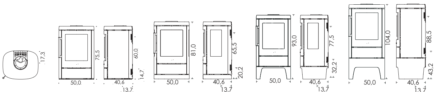
HWAM 4510c met zijruiten en mini sokkel HWAM® Autopilot™
