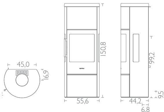
HWAM 3650c met zijruiten
