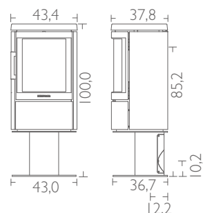
HWAM 2620c met voetstuk
