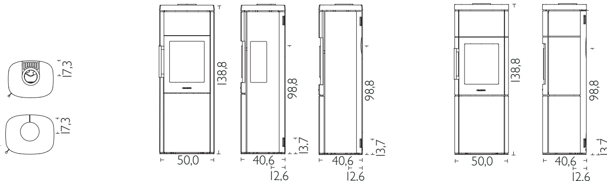
HWAM 4550m met zijruiten
