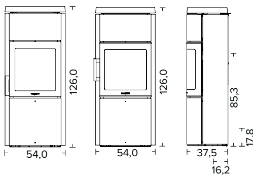
HWAM 3520c met style handgreep, roestvrij staal
