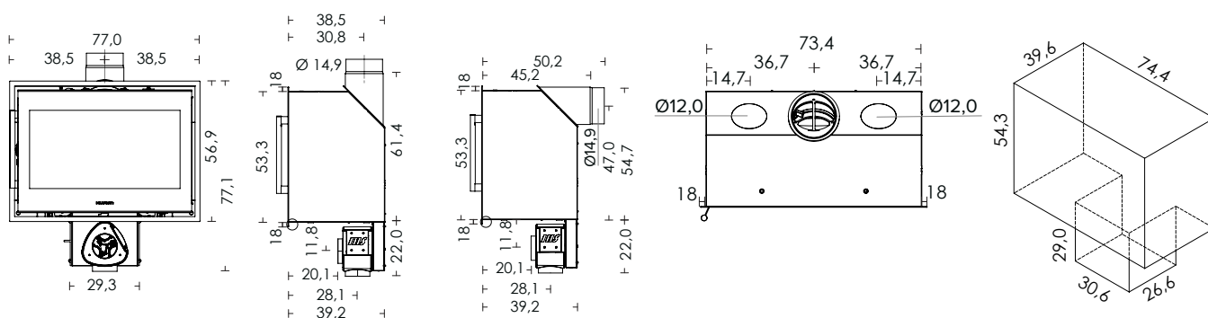
HWAM I 40/55m rechts scharnierend
