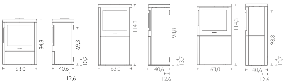
HWAM 4640m met speksteen
