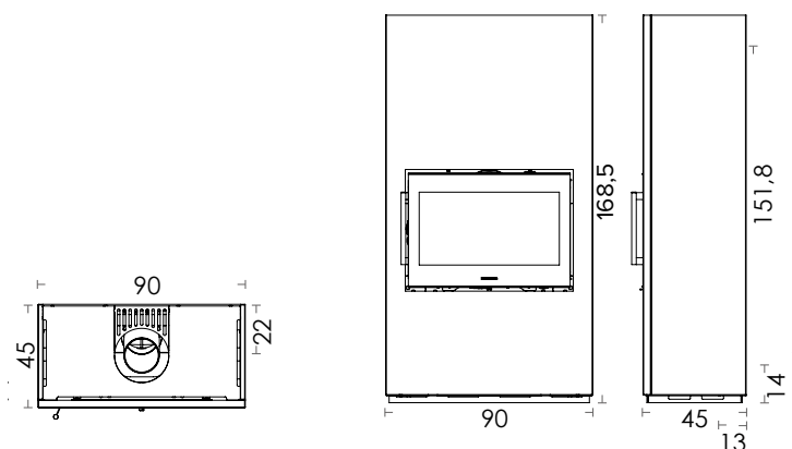
HWAM 5530c, scharnier rechts
