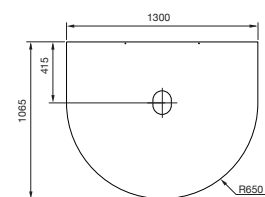
Voor alle modellen met zijruit – Draaihoek 90° Plaatstaal Dikte 1,5 mm, grijs of zwart
