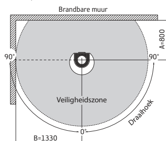
Contura 556, 586 180°, hoek
