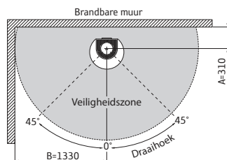
Contura 500 series (niet 556 en 586) 90°, hoek
