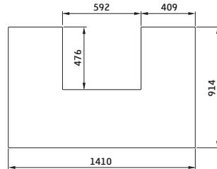
Contura i61-serien Glas Dikte 6 mm
