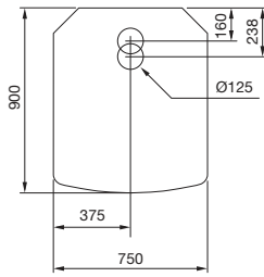
Contura 50-serien Plaatstaal Dikte 1,5 mm
