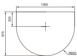
Voor alle modellen zonder zijruit – Draaihoek 90° Plaatstaal Dikte 1,5 mm, grijs of zwart
