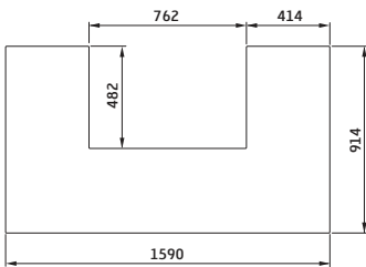
Contura i51-serien Glas Dikte 6 mm
