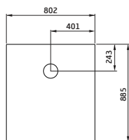
Contura 130 Plaatstaal Dikte 1,5 mm
