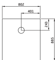
Contura 210 Plaatstaal Dikte 1,5 mm
