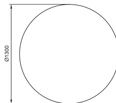
Voor alle modellen – Draaihoek 180°- en 360° Plaatstaal Dikte 1,5 mm, grijs of zwart
