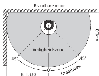
Contura 556, 586 90°, hoek
