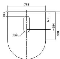
Vloerplaat voor plaatsing onder vrijstaande kachels - alle modellen Plaatstaal Dikte 1,5 mm grijs of zwart
