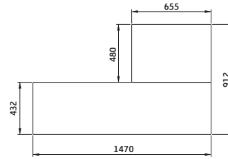
Contura i41-serien, bank Glas Dikte 6 mm
