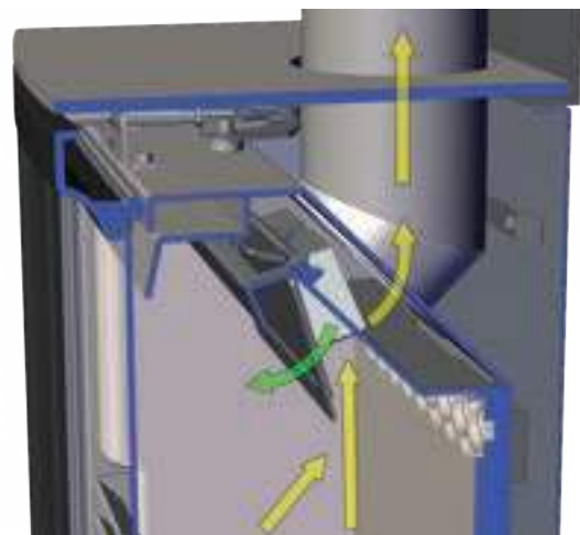
Purevision Actieve Klep Systeem Open
