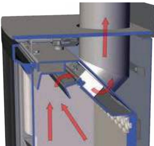
Purevision Actieve Klep Systeem Dicht
